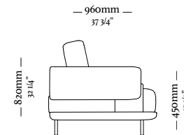
Sofá 3 Lugares c/ 2 br 1870 x 960 x 820mm
