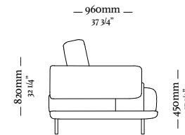
Sofá 3 lugares c/ 1 br 1730 x 960 x 820mm
