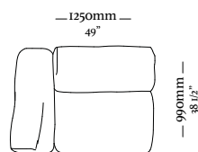
Módulo c 1 br ass. 900 1250 x 990 x 780
