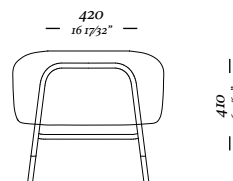
Banqueta 730x420x410 mm
