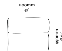
Módulo s/ br ass. 1100 1100 x 990 x 780
