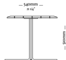
MH 9118 563 x 540 x 510mm
