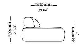
Módulo central Ass. 1150 1150 x 1010 x 750
