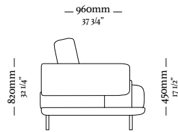
Sofá 1 lugar c/ 1 br 1050 x 960 x 820mm
